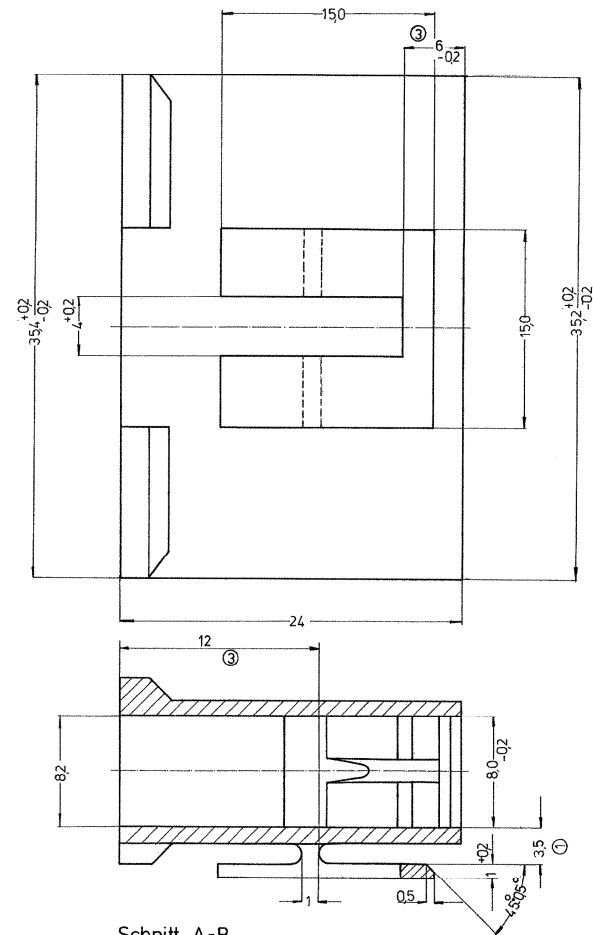
Schnitt A-B
