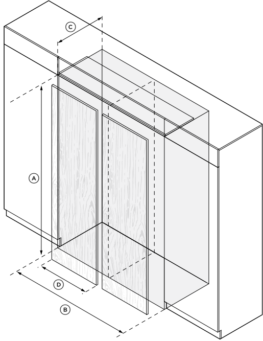
INSTALLAZIONE DOPPIA
