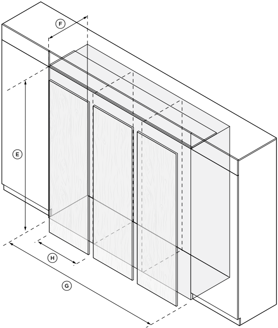
INSTALLAZIONE TRIPLA
