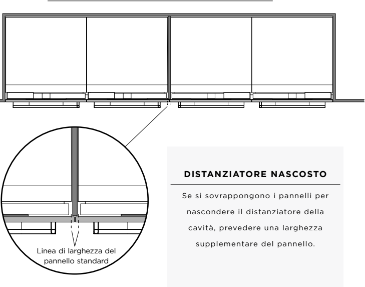
DOPPIA CAVITÀ CON DISTANZIATORE NASCOSTO
