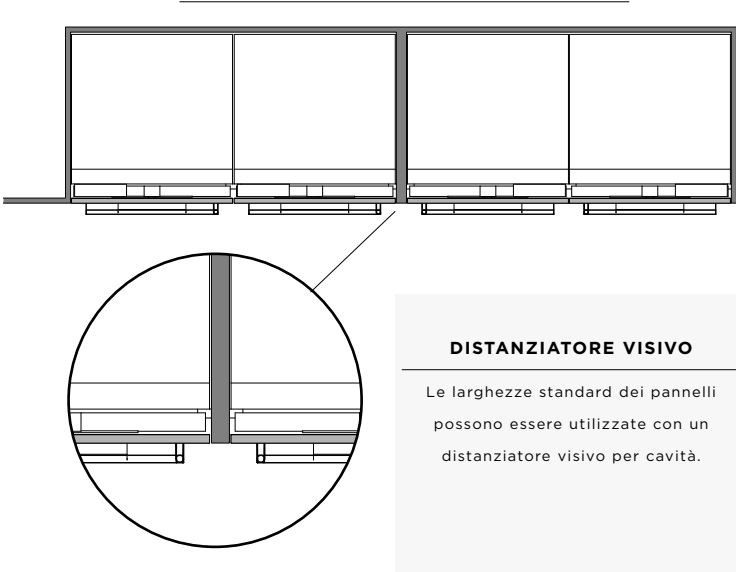
DOPPIA CAVITÀ CON DISTANZIATORE VISIVO
