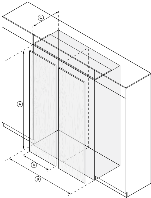
INSTALACIÓN DOBLE
