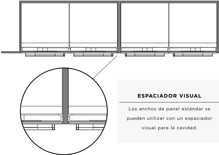
DOBLE CAVIDAD CON ESPACIADOR VISUAL
