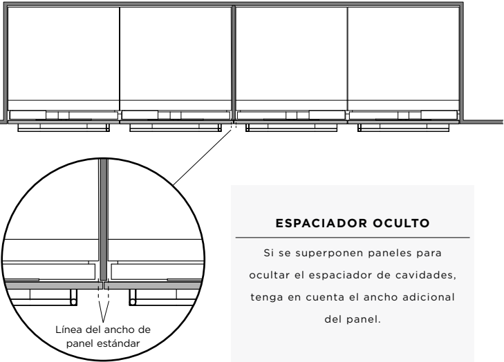
DOBLE CAVIDAD CON ESPACIADOR OCULTO
