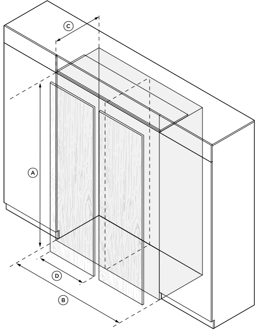
DUBBEL INSTALLATION
