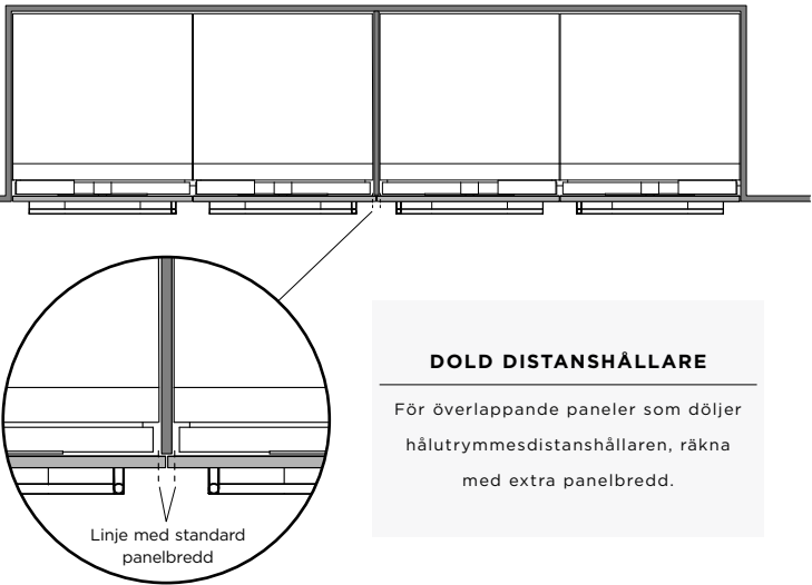
DUBBELT HÅLUTRYMME MED DOLD DISTANSHÅLLARE
