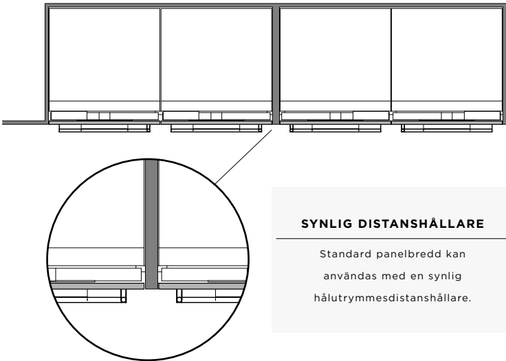
DUBBELT HÅLUTRYMME MED SYNIG DISTANSHÅLLARE
