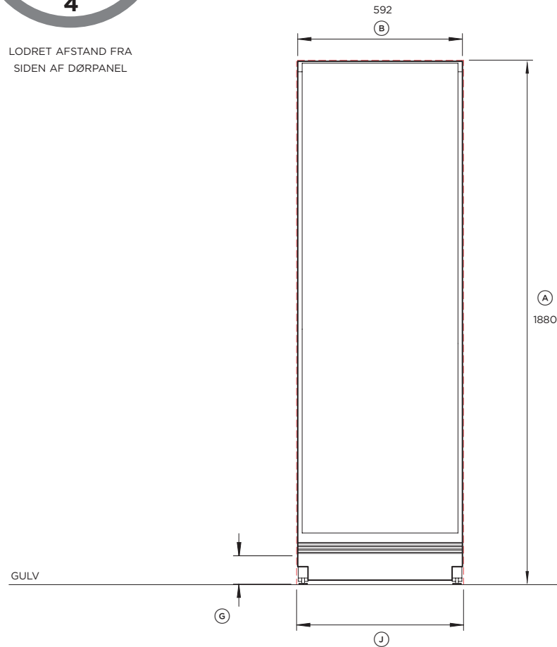
VISNING FORFRA
