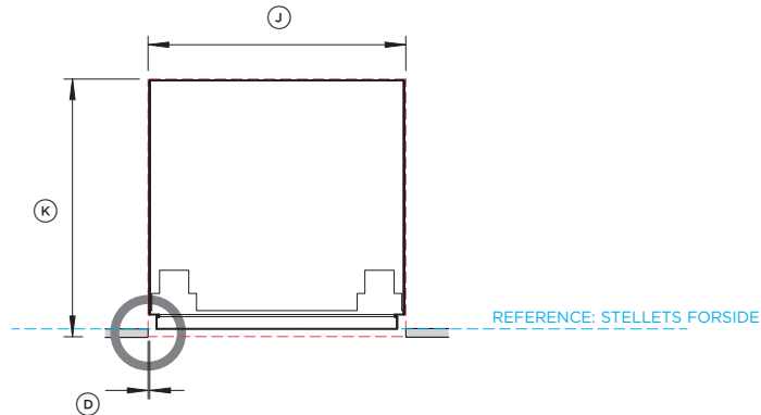
PLANVISNING
