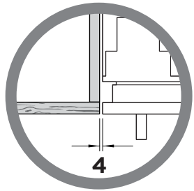
LODRET AFSTAND FRA SIDEN AF DØRPANEL
