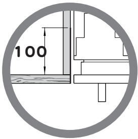
安装柜侧面和顶面回路
