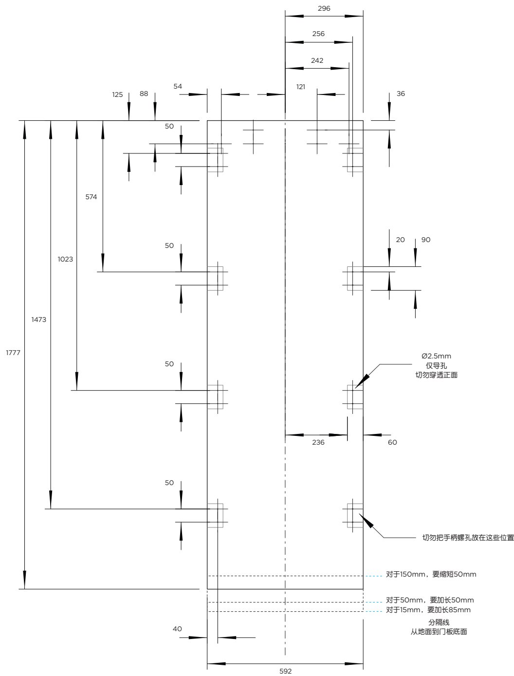
后视图
