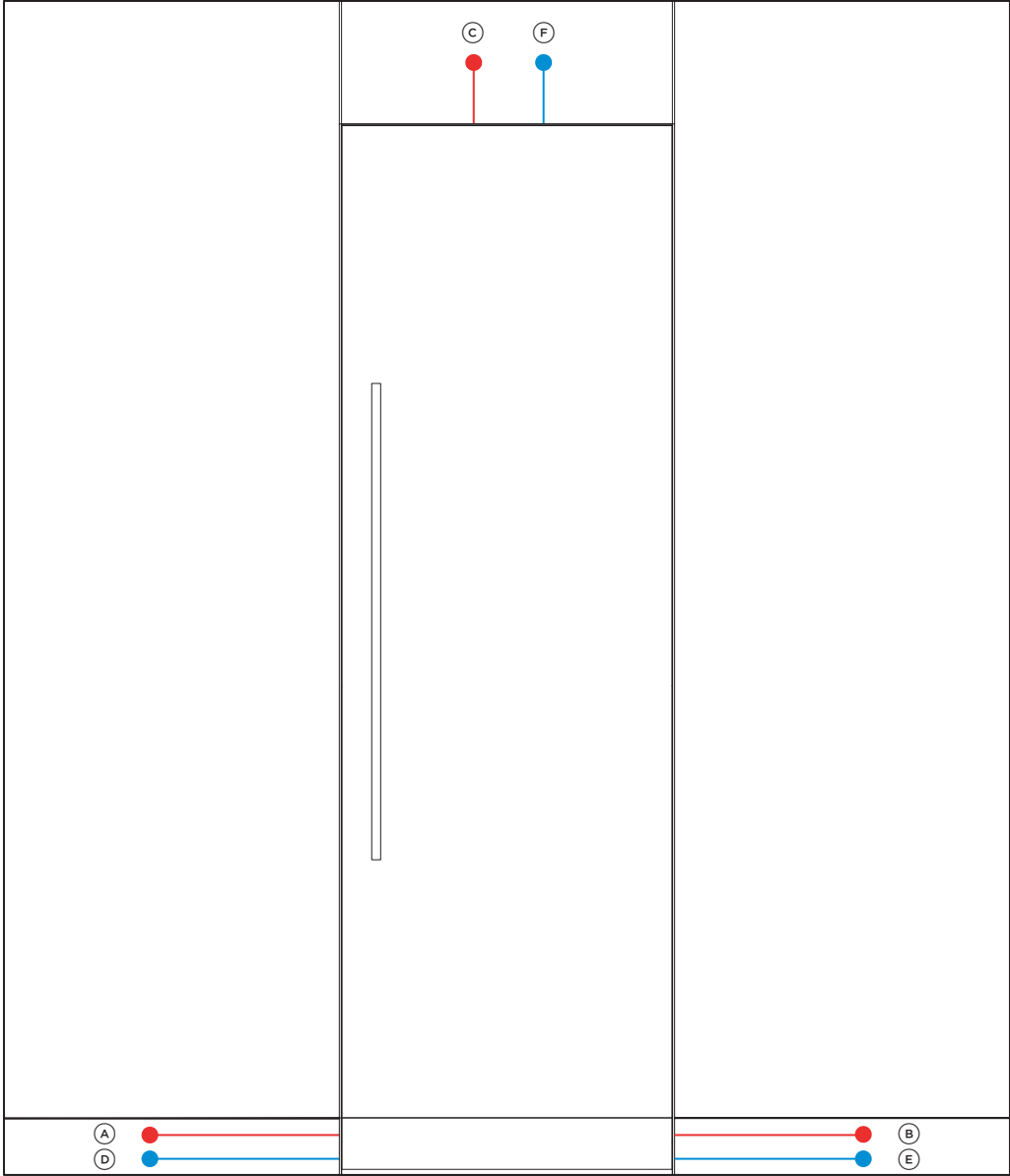
正视图
