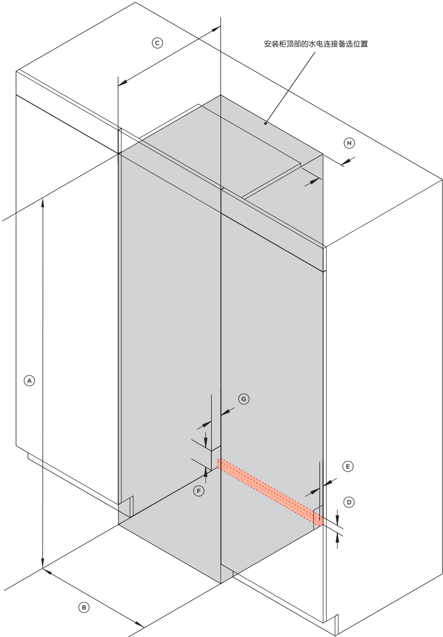
正等轴测图
