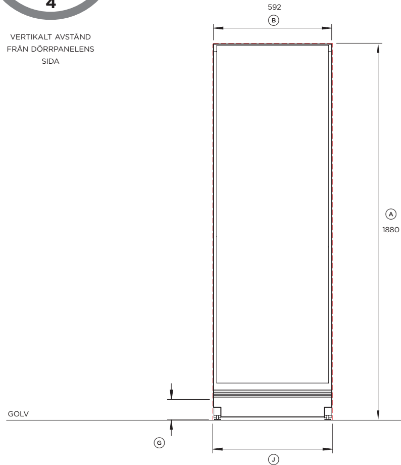
FRONTVY
