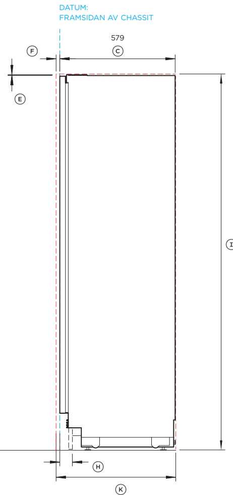
PROFILVY
