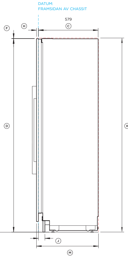
PROFILVY
