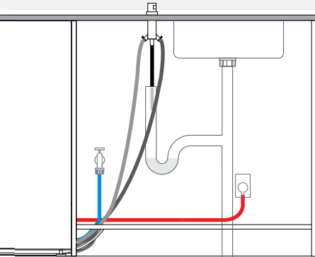
INSTALACIÓN DE ESPACIO DE AIRE DOBLE
