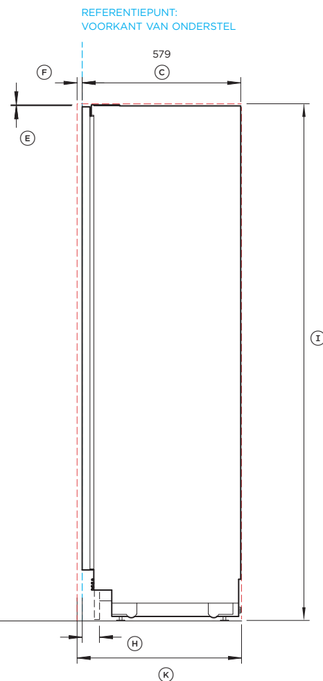
ZIJAAANZICHT
