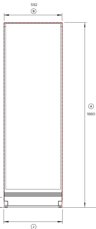
VOORAANZICHT
