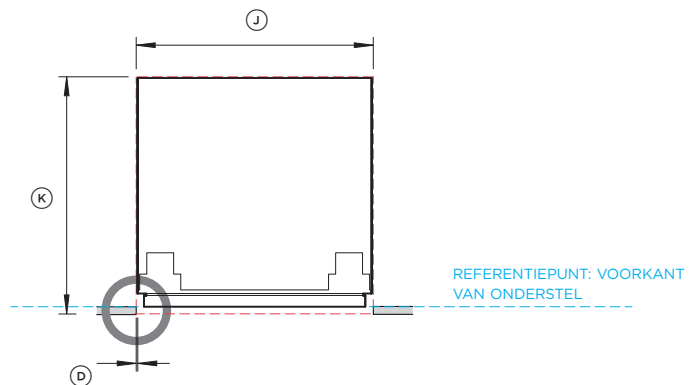
BOVENAANZICHT
