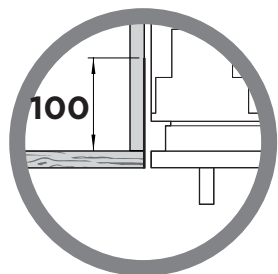
AFWERKINGSPANEEL INBOUWNIS ZIJKANTEN & BOVENKANT
