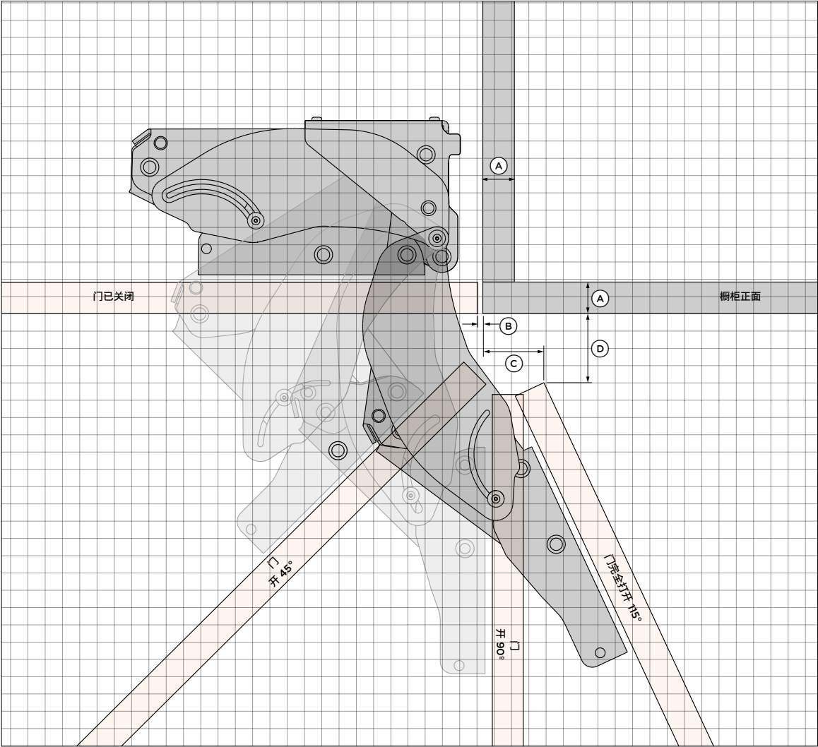
俯视图
