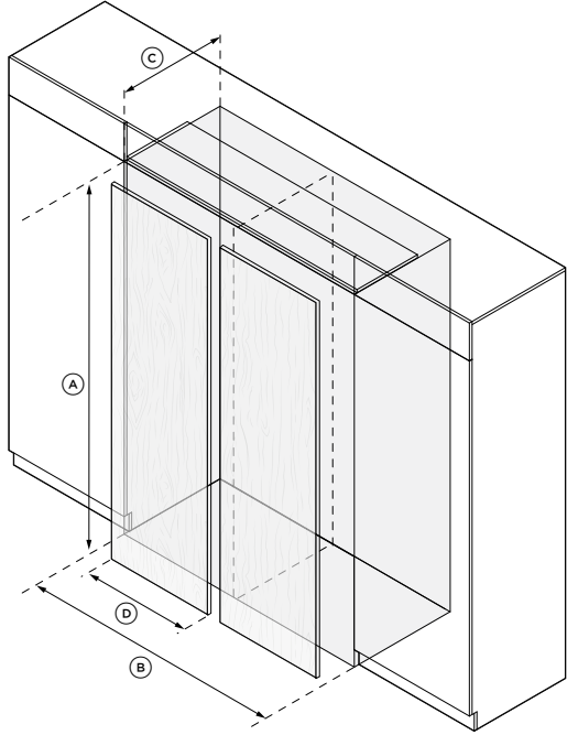
双机安装
