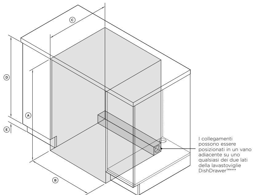
VISTA ISOMETRICA
