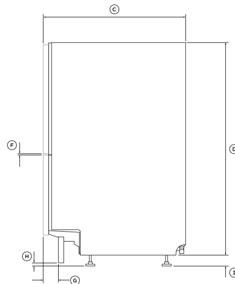
PROFILO
