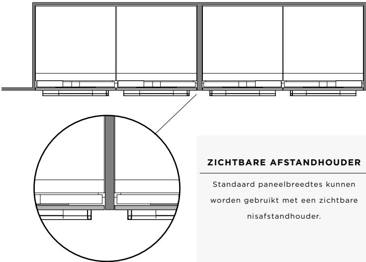
DUBBELE NIS MET ZICHTBARE AFSTANDHOUDER
