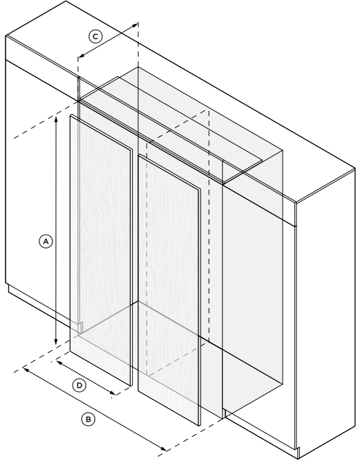
TWEEVOUDIGE INSTALLATIE
