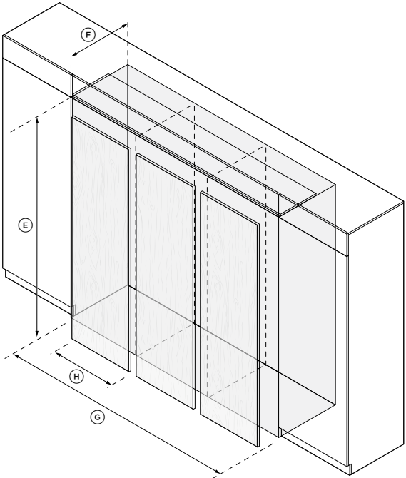
DRIEVOUDIGE INSTALLATIE
