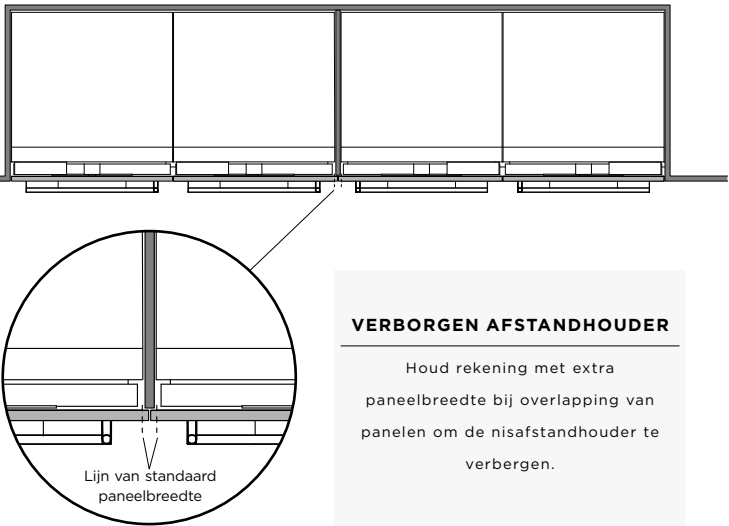
DUBBELE NIS MET VERBORGEN AFSTANDHOUDER
