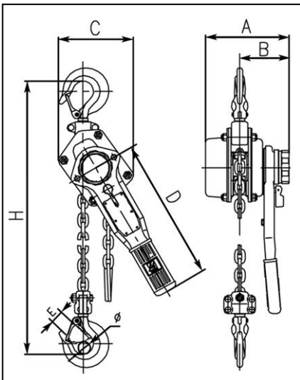
Fig. 1 Målskisse
