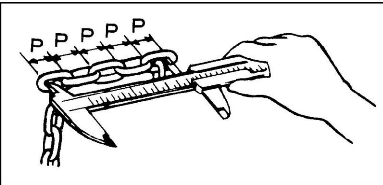
Kuva 7 Ketjun kontrollimittaus
