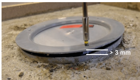
8. Justera till önskad höjd, max 15 mm. Glipan mellan fläns och brunn behöver vara minst 3 mm så att flytspackel kommer in. OBS! Skruvarna får endast justeras med handverktyg.
