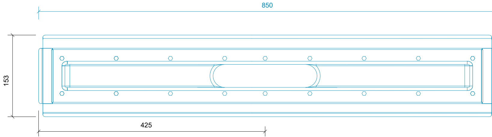
Plan/Plan/Draufsicht
