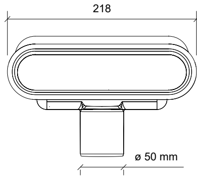
Plan/Plan/Draufsicht
