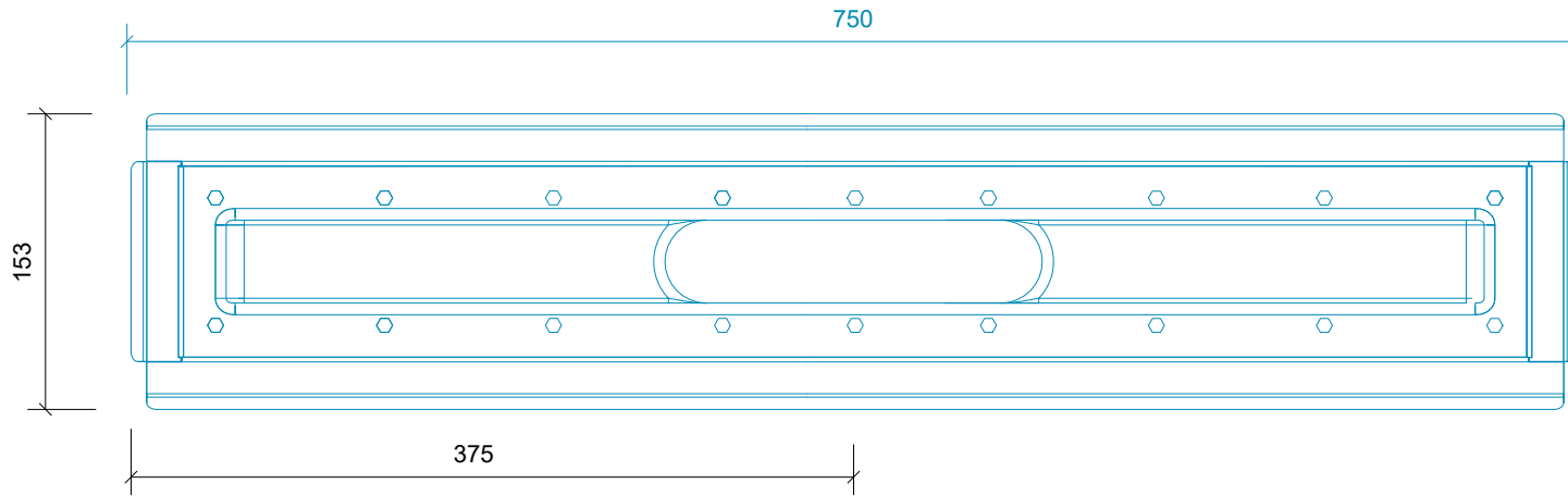
Plan/Plan/Draufsicht
