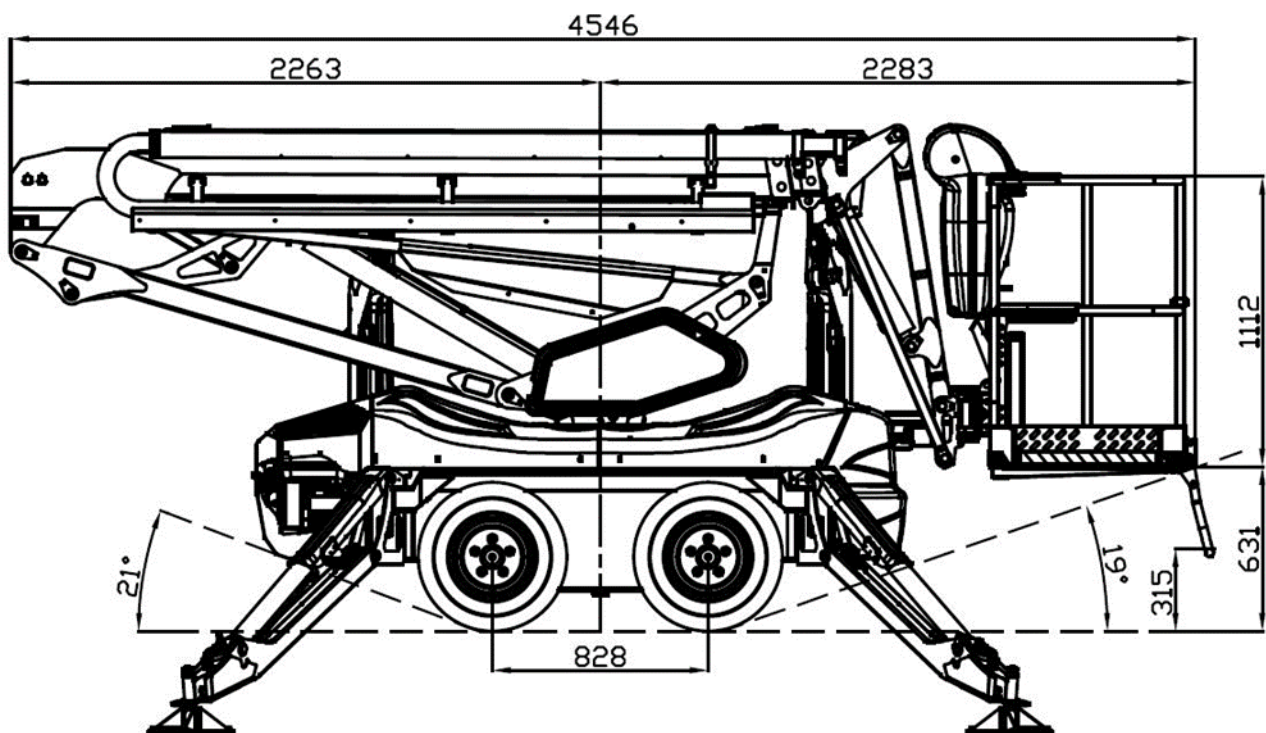
Kuva 2 Päämitat, sivu
