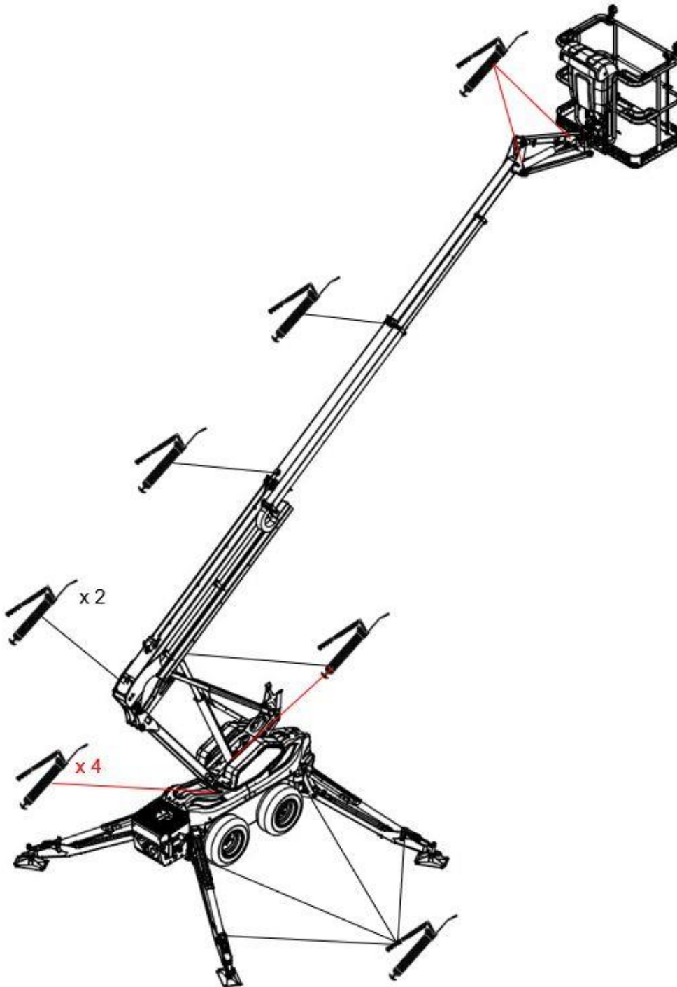
Kuva 14 Voitelukaavio
