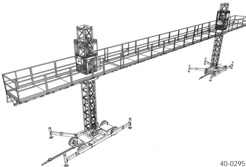
Kuva 1.4. SC4000 kaksimastolava pyörialustalla.
