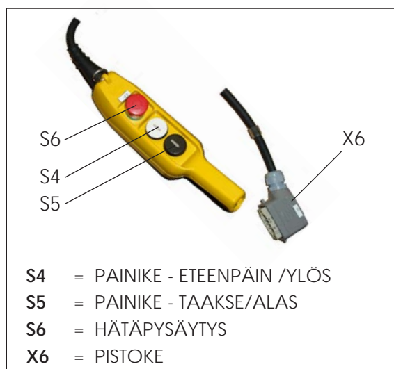
Kuva 4.15. Kauko-ohjain E3 (vaakasuora ja pystysuora ajo).
