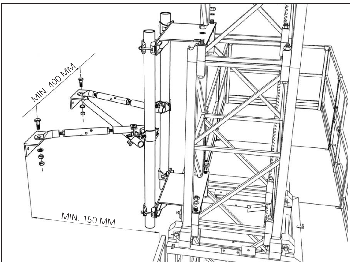
Kuva 4.6. Pystysäätöankkuri.
