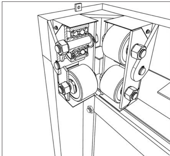
Kuva 6.9. Ohjausrullat.
