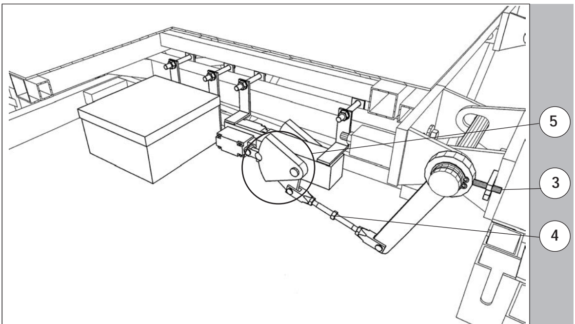
Kuva 4.35. Tasauslaitteen säätö.
