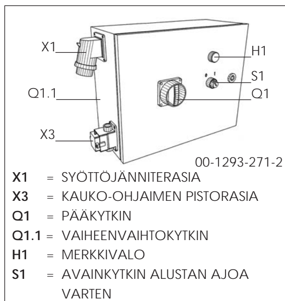
Kuva 4.14. Alustan sähkökaappi.
