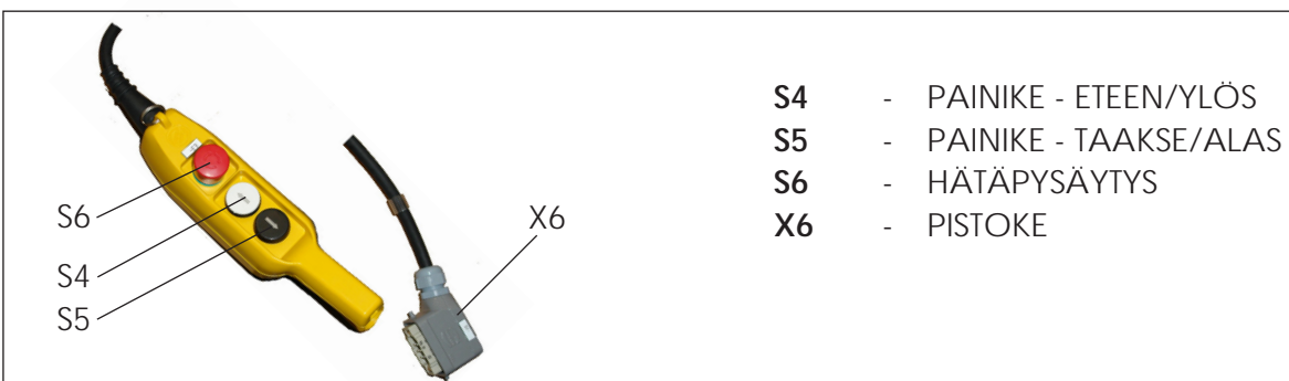
Kuva 5.3. Kauko-ohjain E3 (vaakasuora ja pystysuora ajo).
