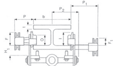
Malli HTP 500 - 5000 kg lukituslaitteella
