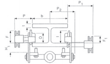
Malli HTG 500 - 5000 kg lukituslaitteella
