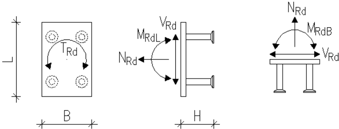
Kuva 3. SBKL-kiinnityslevyjien voimien suuntien merkinnät
