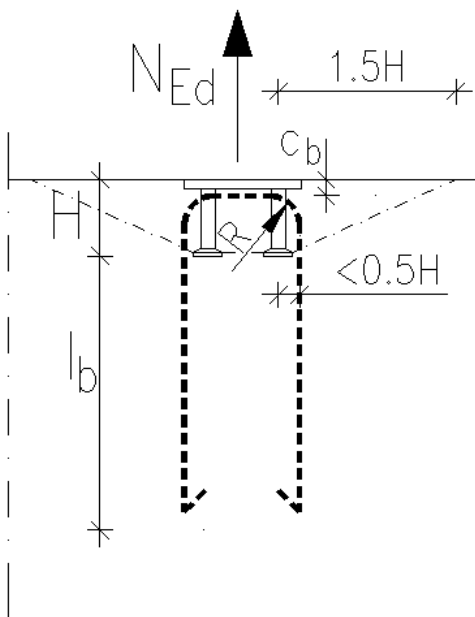
Kuva 6. SBKL-kiinnityslevyn lisäraudoitus vetokestävyydelle ja taivutusmomenteille
