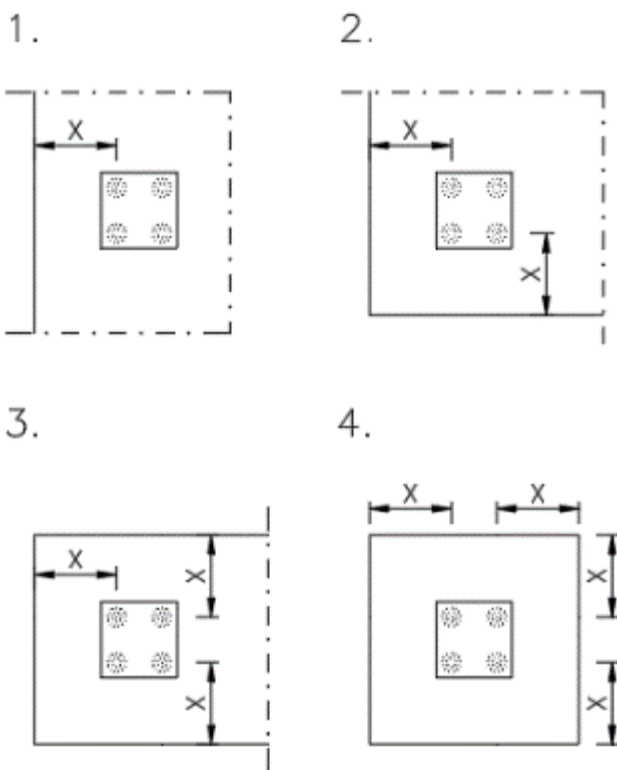
Kuva 1. Reunaetäisyyksien merkinnät (1-4 reunaa)
