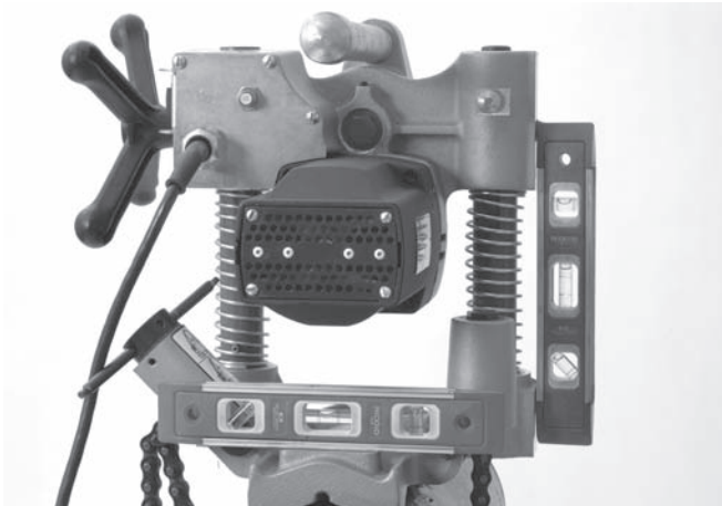
Şekil 10 – HC-300 Düzleme
