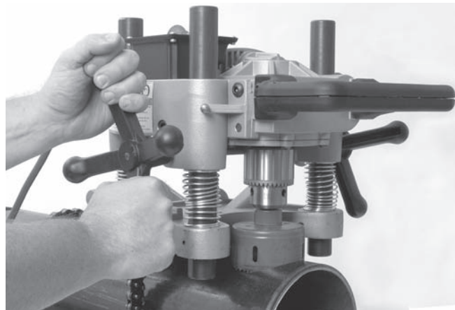
Kuva 11 – Reikäsahauslaitteen käyttö
