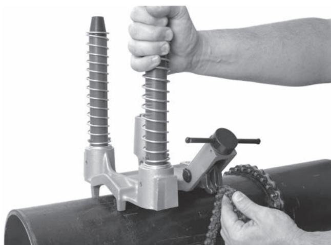
Rysunek 8 – Zahaczanie łańcucha
