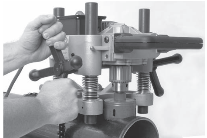
Figur 11 – Bruke hullemaskinen
