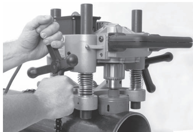
Figur 11 – Använda håltagningsverktyget
