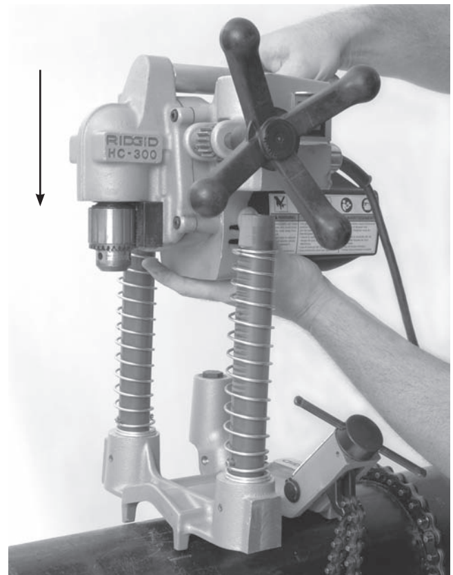
Slika 9 – Spajanje HC-300 motornog sklopa na bazni sklop
