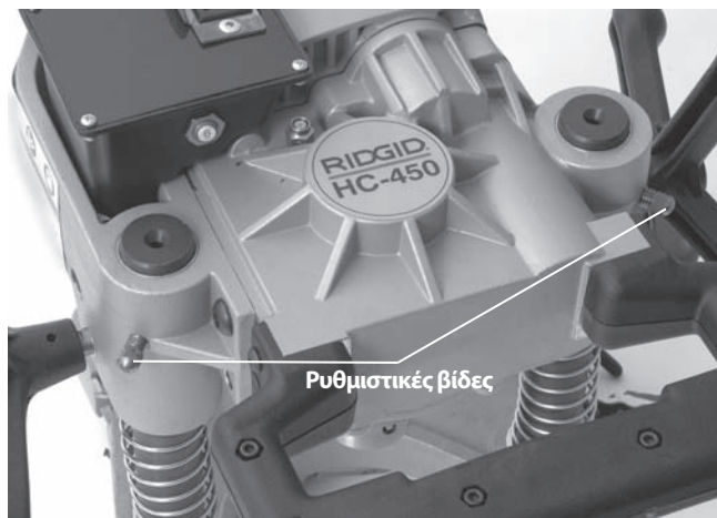
Εικόνα 13 – Προσαρμογή των ρυθμιστικών βιδών
