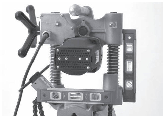
Kuva 10 – HC-300:n oikaisu
