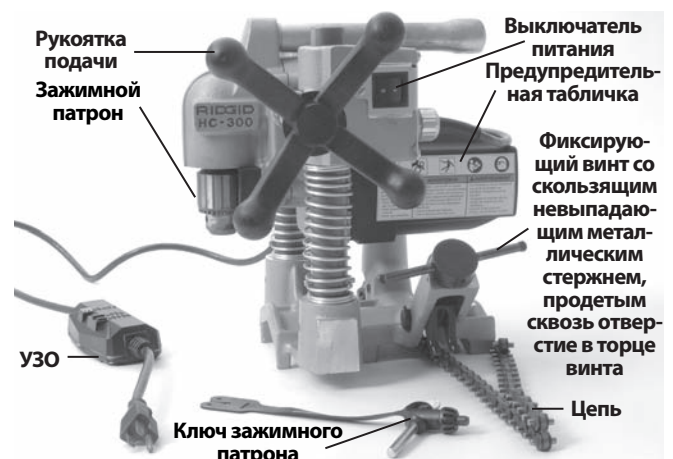
Рис. 2 – Модель HC-300 со стандартными принадлежностями
