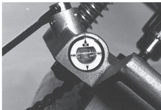
Figur 6 – HC-450 Håltagningsverktygets vattenpass
