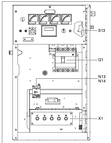
Q1..... Huvudströmbrytare
