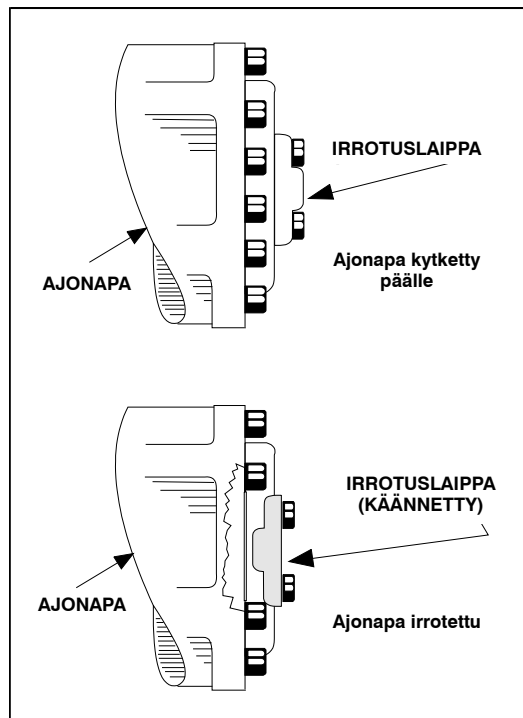
Kuva 4-4. Ajon irrotusnapa
