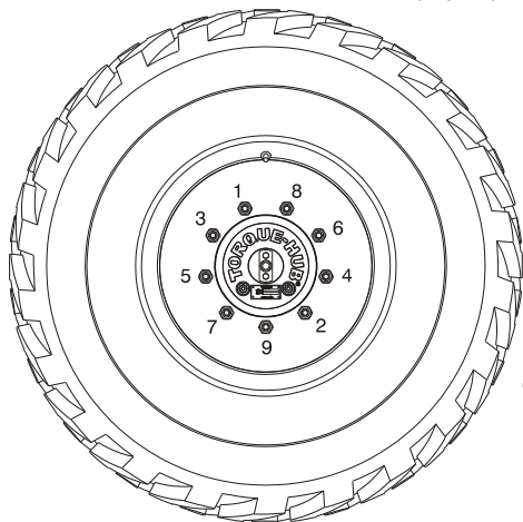
9 MUTTERIKUVIO
