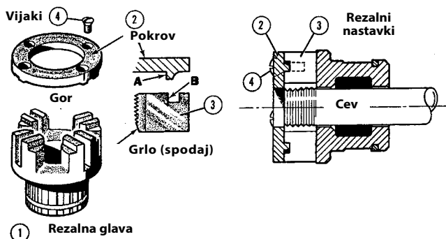
Slika 17 – Vgradnja rezalnih nastavkov v glavo
