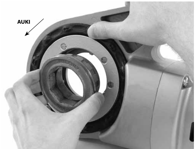
Kuva 8 – Välikappaleen asennus 690-I:een
