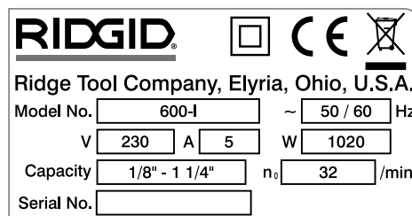
Abbildung 4 - Geräteseriennummer
