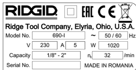
Slika 4 – Serijska številka naprave
