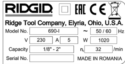
Figur 4 – maskinserienummer
