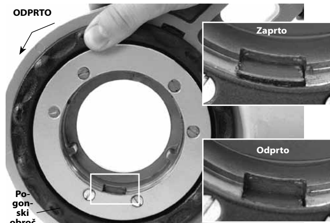
Slika 7 – Držalni mehanizem, pogonski obroč v odprtem/zaprtom položaju
