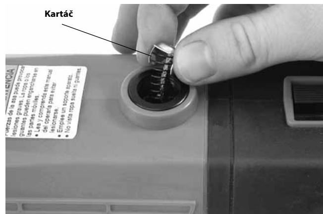
Obrázek 18 – instalace kartáče
