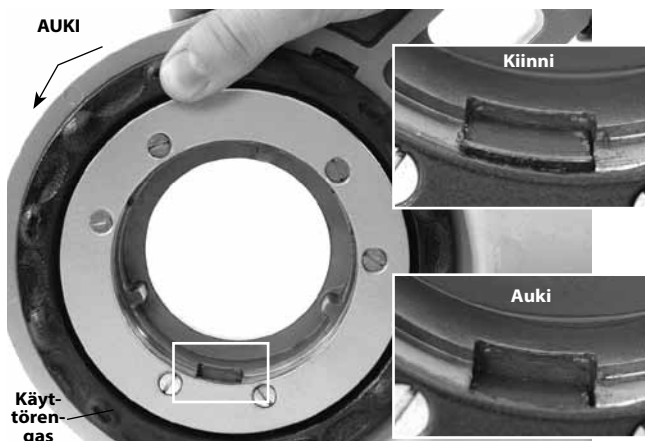
Kuva 7 – Kiinnitysmekanismi, käyttörengas auki-/kiinni-asennossa
