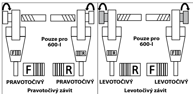
Obrázek 10 – posuvný spínač/orientace závitorezné hlavy
