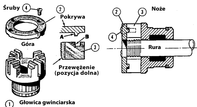
Rys. 17 – Zakładanie noży do głowicy
