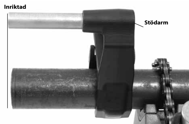
Figur 11B – Inställning av stödarmen
