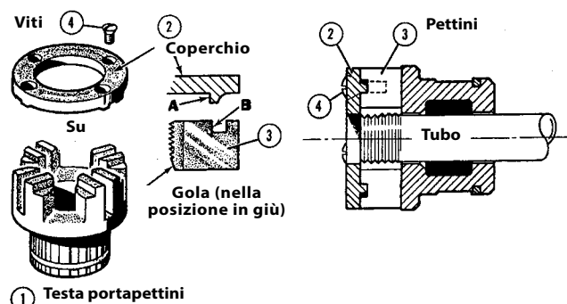
Figura 17 – Installazione dei pettini nella Testa portapettini
