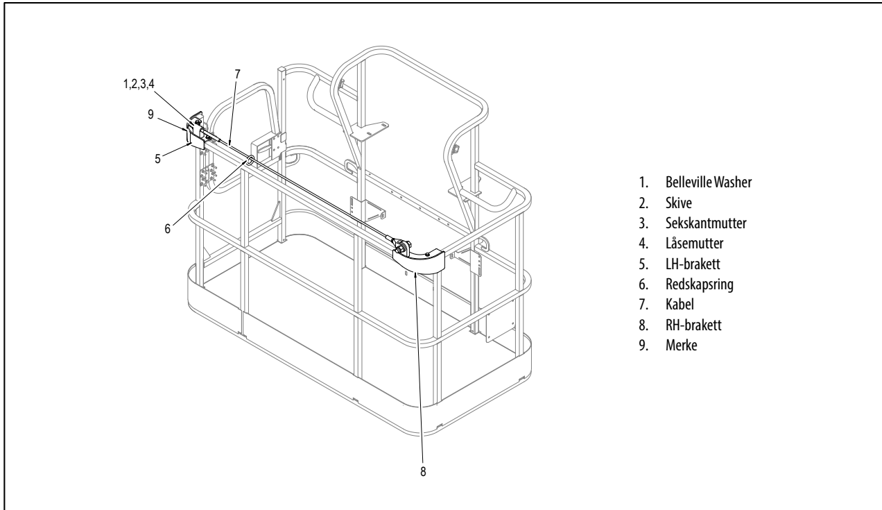
Figur 6-3. Eksternt "bolt-på"-fallsikringsystem
