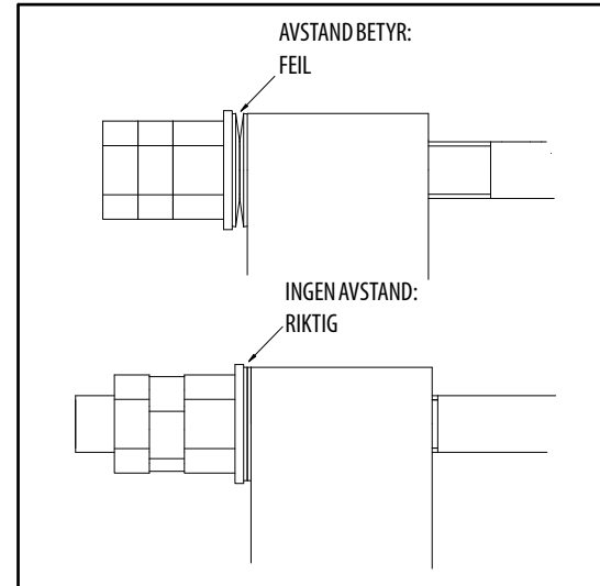
Figur 6-2. Stramming av kabel i det eksterne "bolt-på"-fallsikringssystemet
