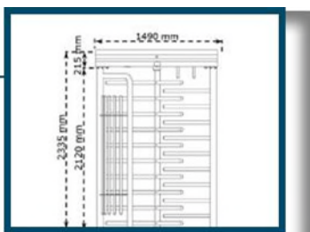
Ritning med mål. Passagehöjd är 2m. Passagebredden 0,6m.
