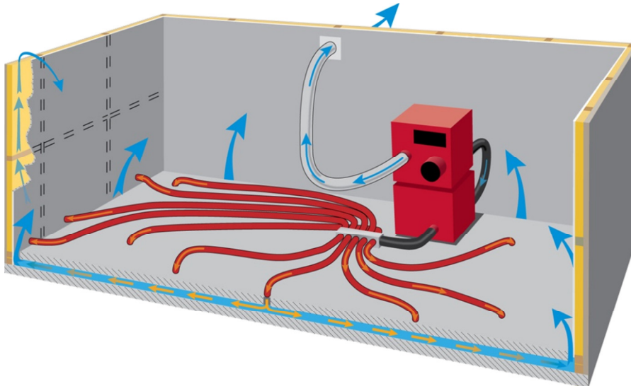
Puhalluskuivaus. Turbiini ottaa kuivailmaa suoraan tilakuivaimesta (CTR 300XT) 50mm:n letkukytken avulla, ja ohjaa sitä eristetilalliseen rakenteeseen.
