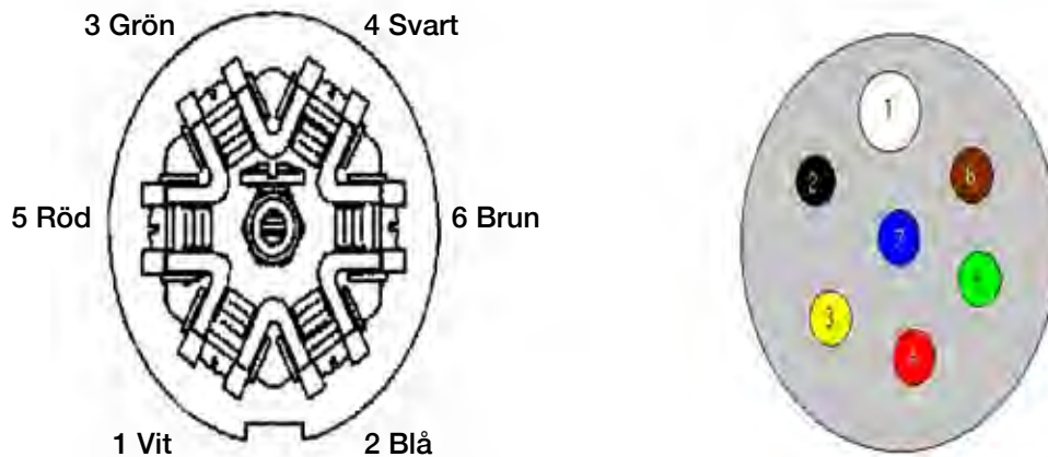
BILD 4: KOPPLINGSSCHEMA FÖR RV- OCH LASTBILSKONTAKTEN
