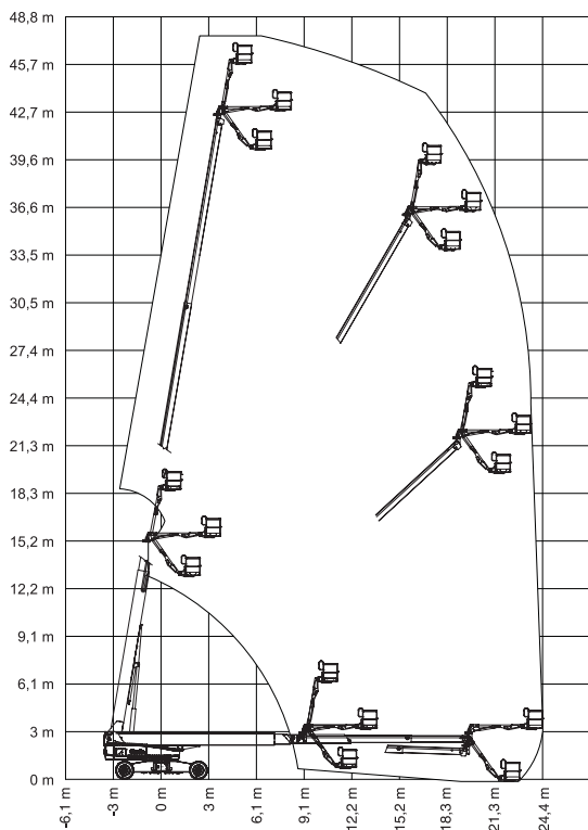
SX-150 liikealuekaavio
