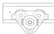
Malli HTG 500 - 5000 kg lukituslaitteella
