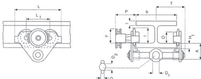
Malli HTG 500 - 5000 kg
