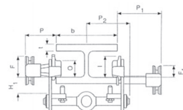
Malli HTG 500 - 5000 kg lukituslaitteella
