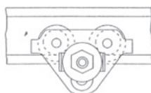
Malli HTP 500 - 5000 kg lukituslaitteella
