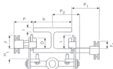
Malli HTP 500 - 5000 kg lukituslaitteella
