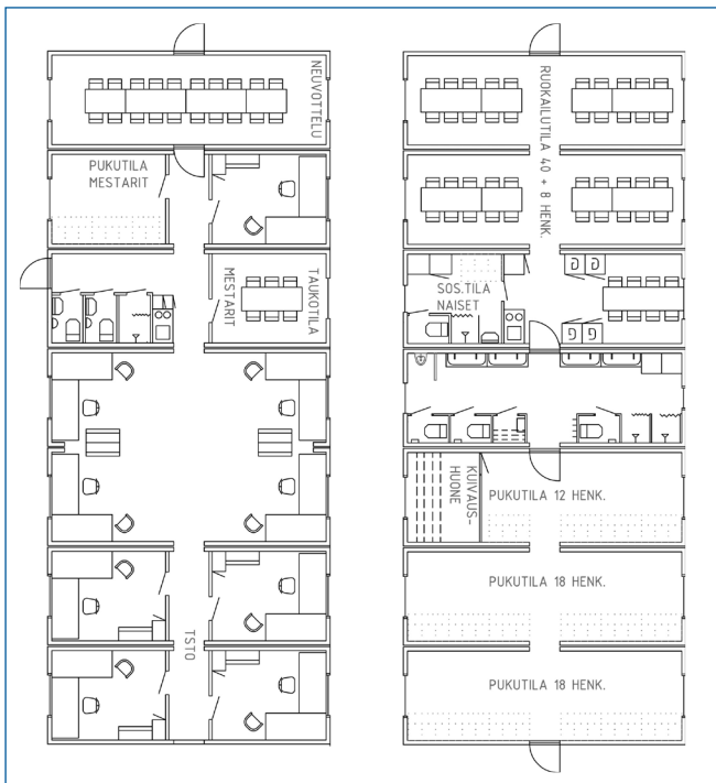
Rami-wood tilojen pohjaratkaisu
