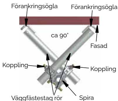
Exempel på förankring som kan uppta horisontalkrafter (OBS! använd typkontrollerade kopplingar)
