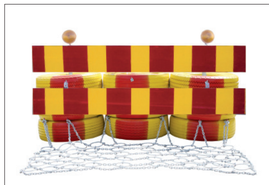
701 1716 X2 Markeringsskärm övre 701 1717 X2 Markeringsskärm nedre Utmärkning för tvärgående avstängning.
