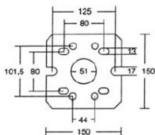
Säätoruuvien levy
