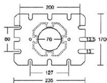
Päätylevy
