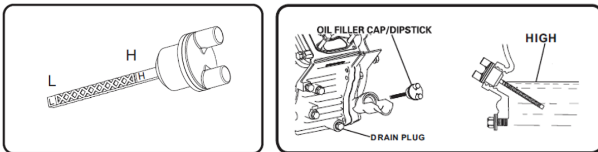
Fig. 9-3 Oljesticka
