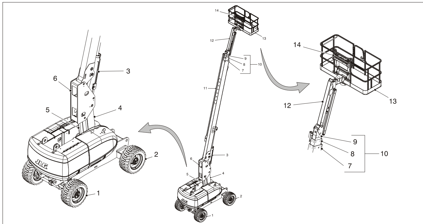
Kuva 2-1. Perusosat - Sivu 1 / 2
