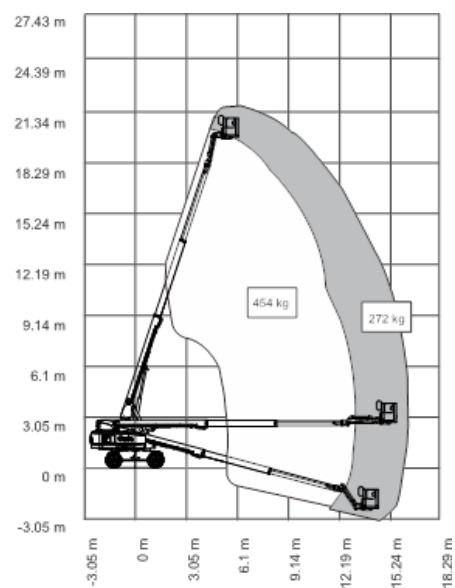
S-65 HF Diagram över rörelseområde
