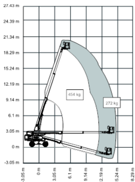
S-65 HF Diagram över rörelseområde
