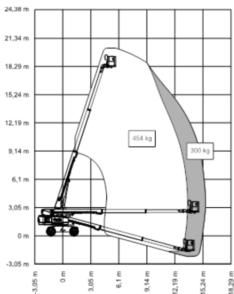
S-65 XC och S-65 TRAX rörelseområde
