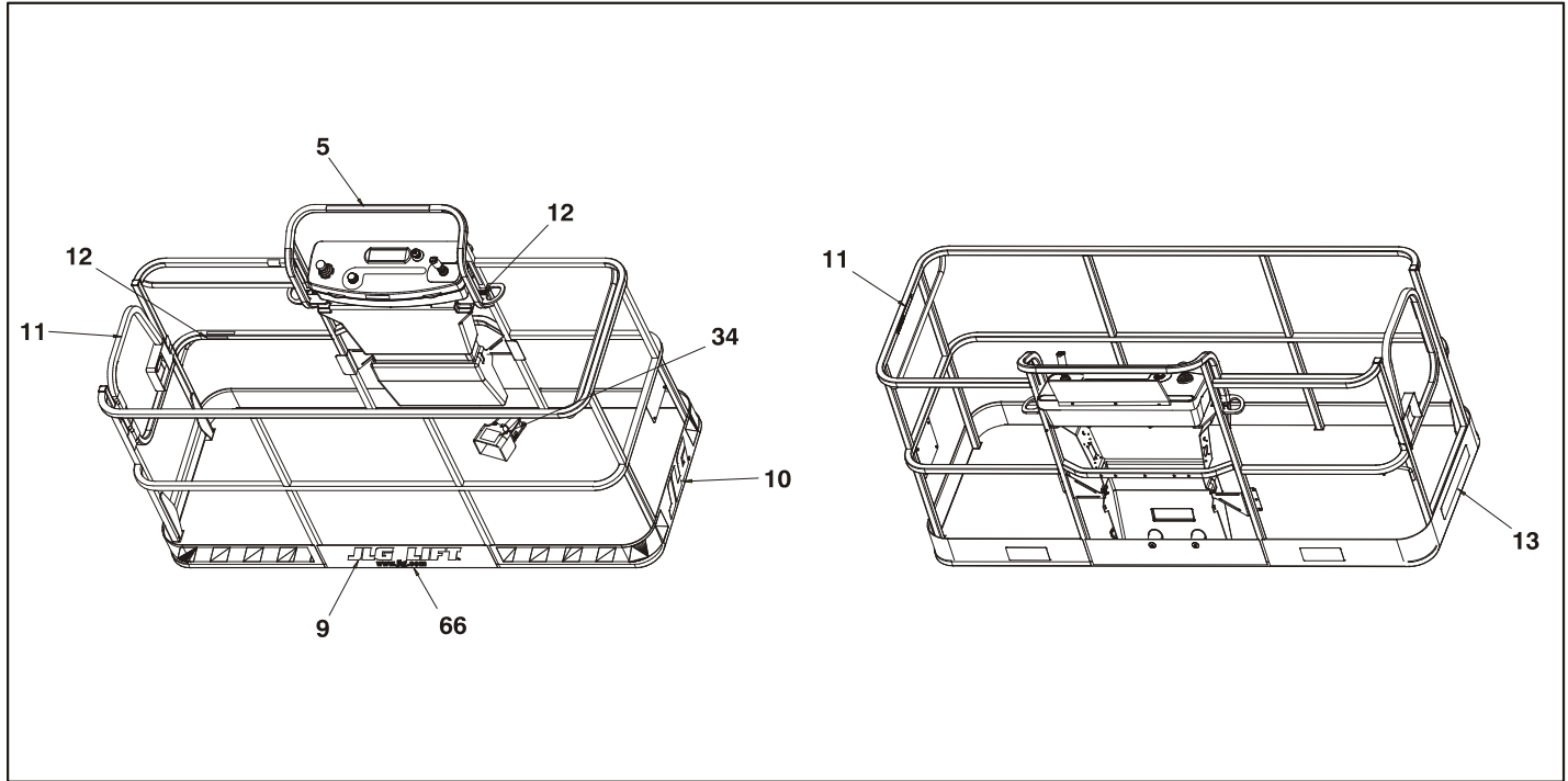
Fig. 4-9. Placering av dekaler – Blad 4 av 4
