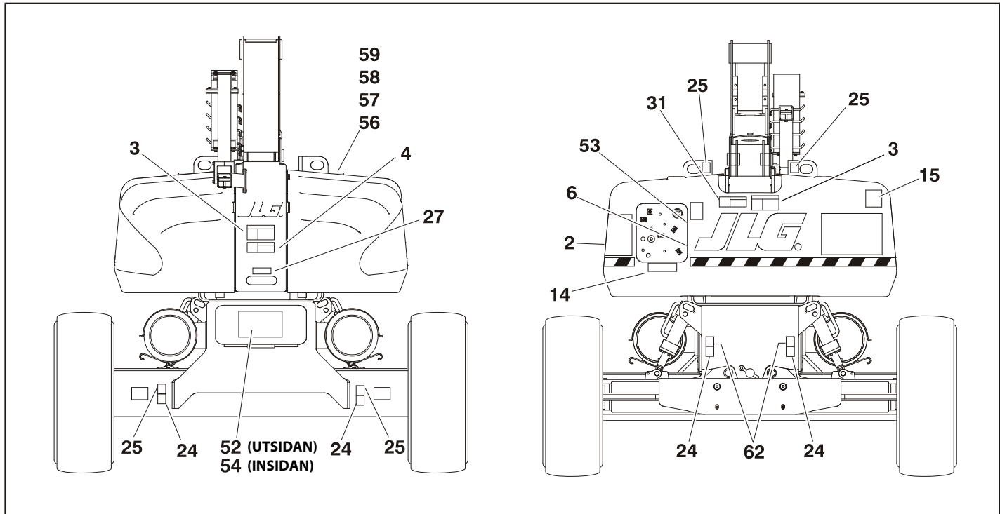
Fig. 4-7. Placering av dekaler – blad 2 av 4
