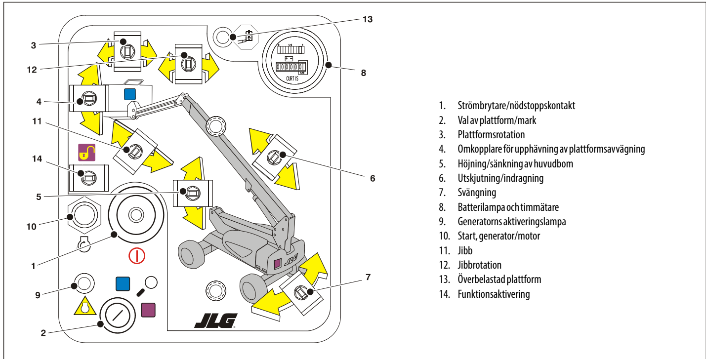
Fig. 3-2. Markpanel med iståndsättning av funktioner
