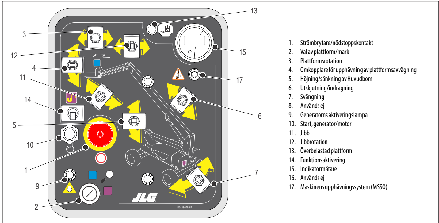
Fig. 3-4. Markpanel med upphävningssystem (MSSO) (endast CE) – serienr 0300202137 tills nu
